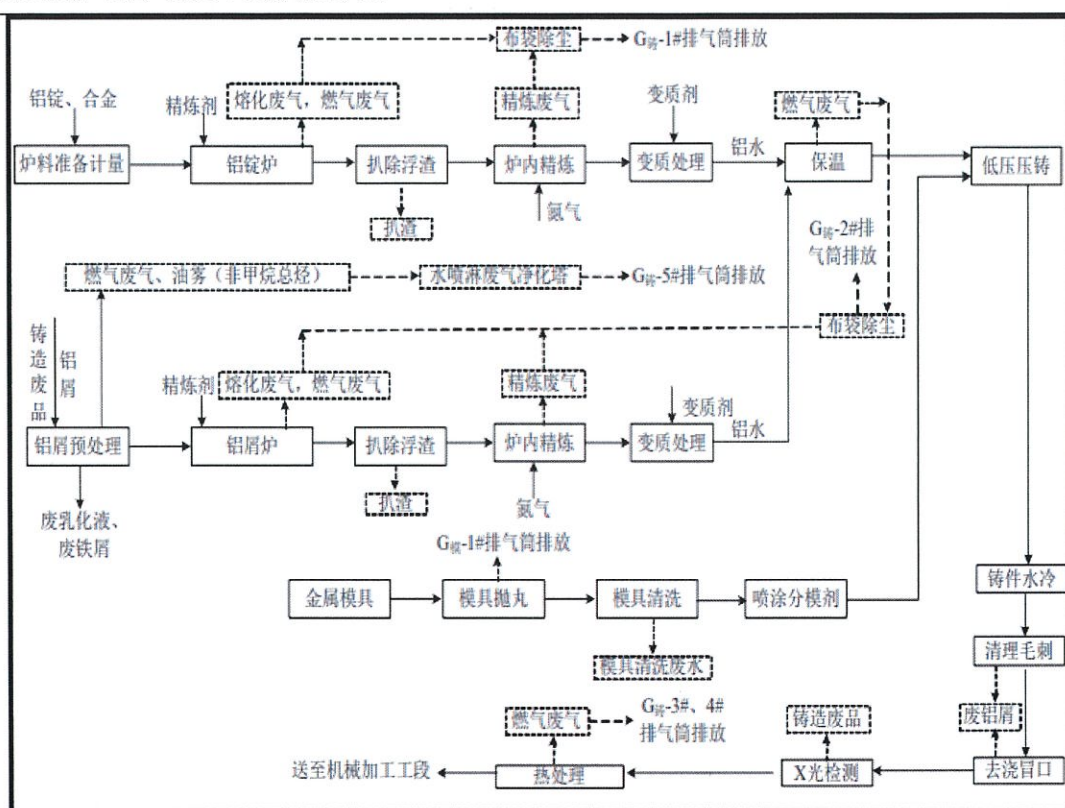
图 3-1-2 铸造车间工艺流程及产污环节示意图
